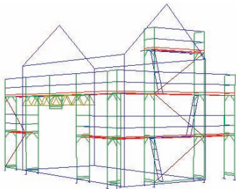
3D-Darstellung eines Fassadengerüsts
