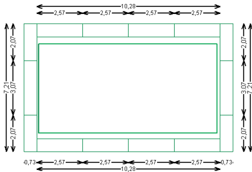
Grundriss eines Fassadengerüsts
